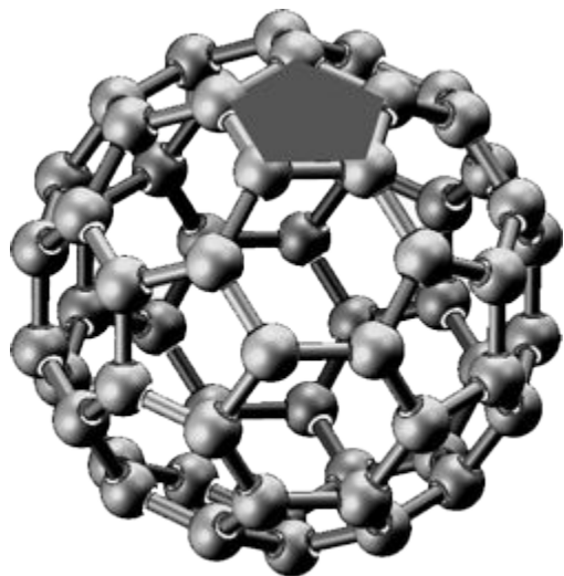
Fullerenenmolekül
